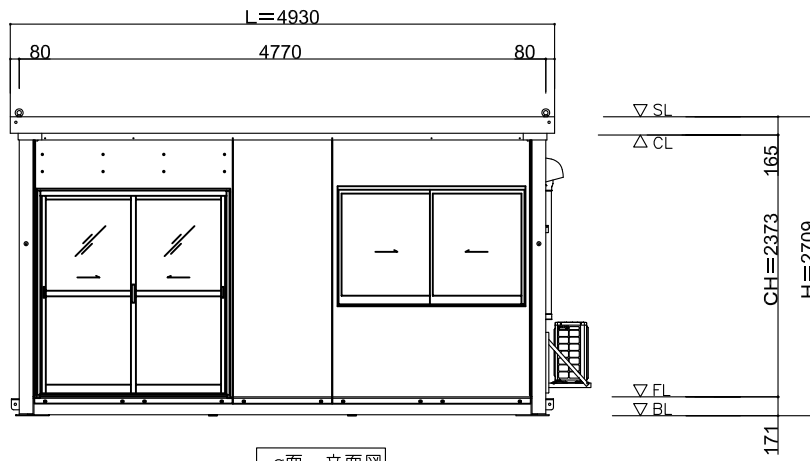
a面 立面図
