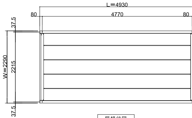
屋根伏図
